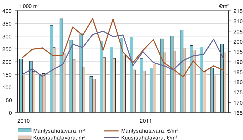
Kuva 1. Suomen mänty- ja kuusisahatavaran vienti (m 3 ) ja viennin yksikköarvot (€/m 3 ), 2010:1–2011:9 (Tullihallitus ja Metla).
