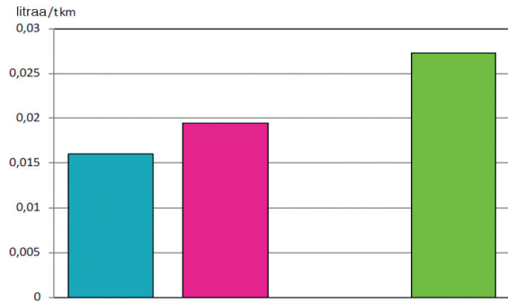
Kuva 5. Polttoaineen kulutus tonnikipometriä kohti. Vertailussa ETT-auto (vasemmanpuoleinen pylväs), tavanomainen puutavara-auto samalla reitillä (keskimmäinen pylväs) ja tavanomaisten puutavara-autojen keskiarvo Ruotsissa (oikeanpuoleinen pylväs) (kuva: Löfroth ja Svenson 2012).
